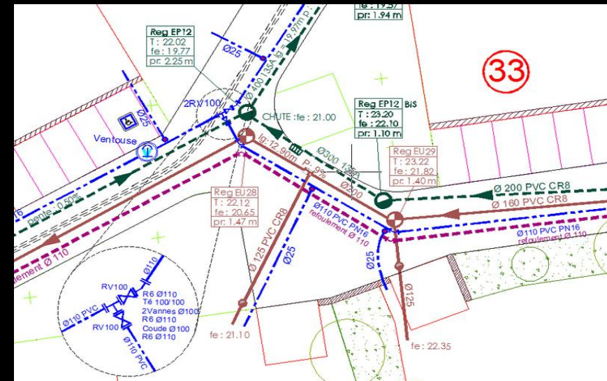
Plan de recollement du réseau d'assainissement
