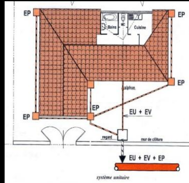
réseau unitaire (tout à l'égout) . موحّد .
