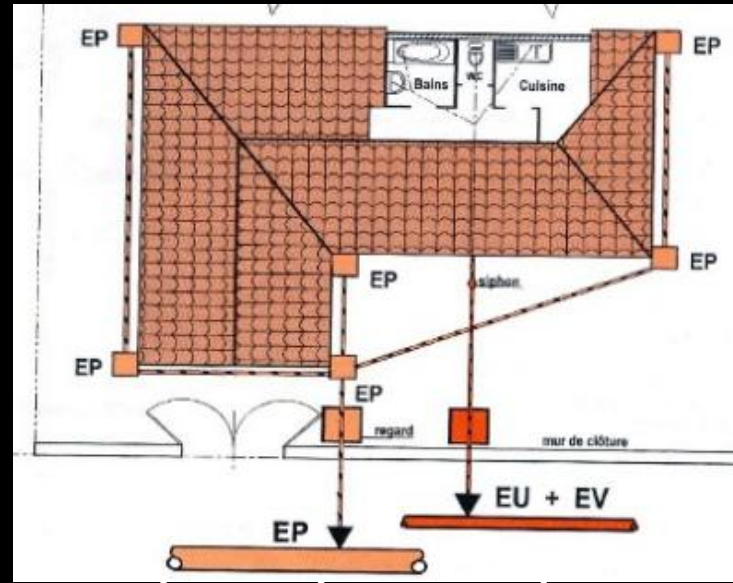
réseau séparatif فردي
