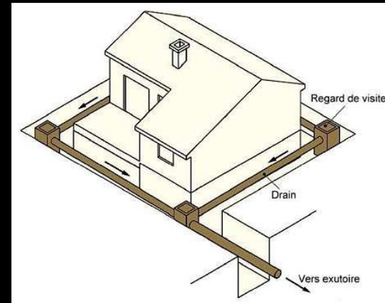
Drain périphérique تصريف محيطي
