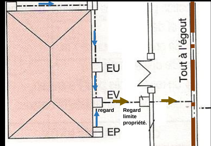
Réseau d'assainissement extérieur unitaire.
